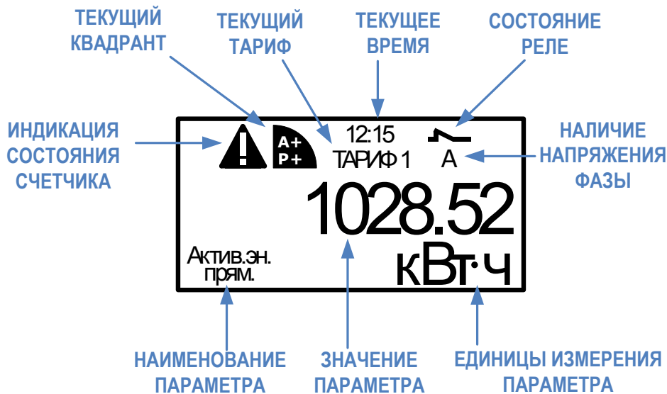
Рисунок 7.4 – Дисплей счетчика для установки на DIN-рейку (тип 3)
