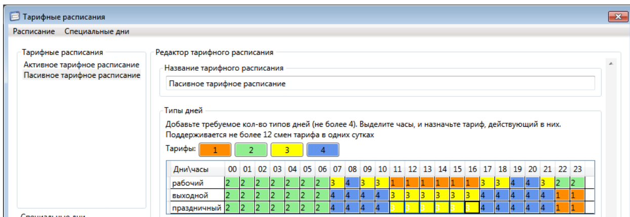
Рисунок 9.35 – Создание нового тарифного расписания
