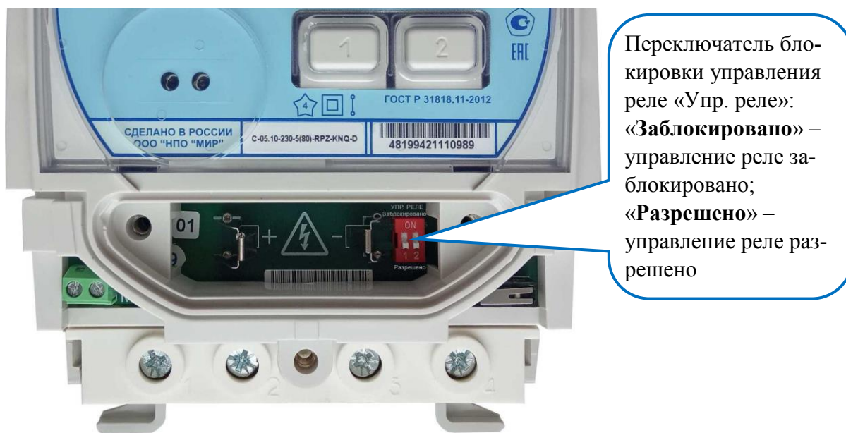
Рисунок Б.7 – Счетчик для установки на щит со снятой крышкой батарейного отсека
