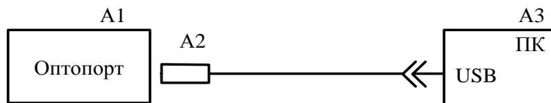
Рисунок В.4 – Схема подключения счетчика в сеть PLC
