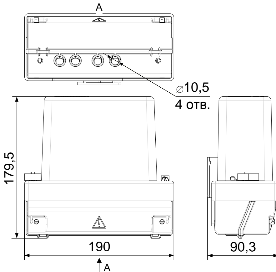
Рисунок Б.4 – Внешний вид, габаритные и установочные размеры счетчика наружной установки
