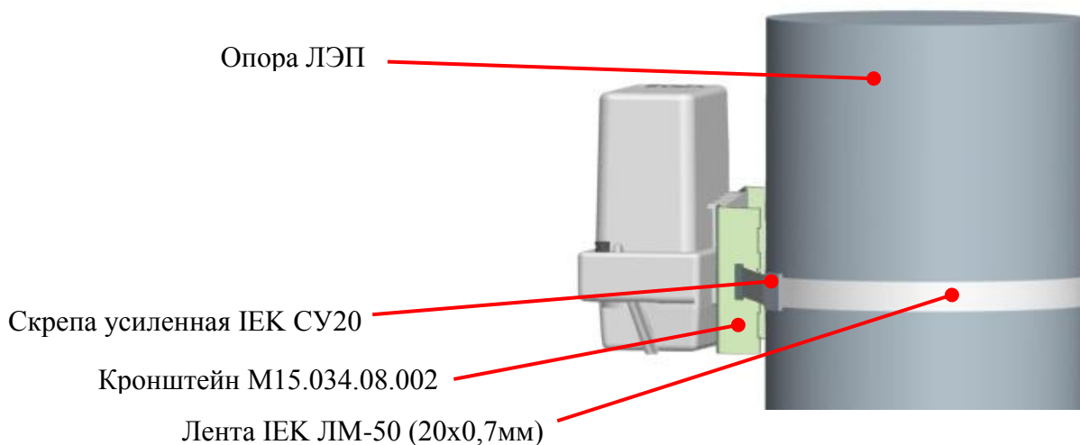
Рисунок 9.3 – Установка счетчика на опору ЛЭП
