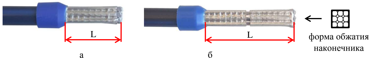
Рисунок 9.1 – Пример обжатия многожильного провода
