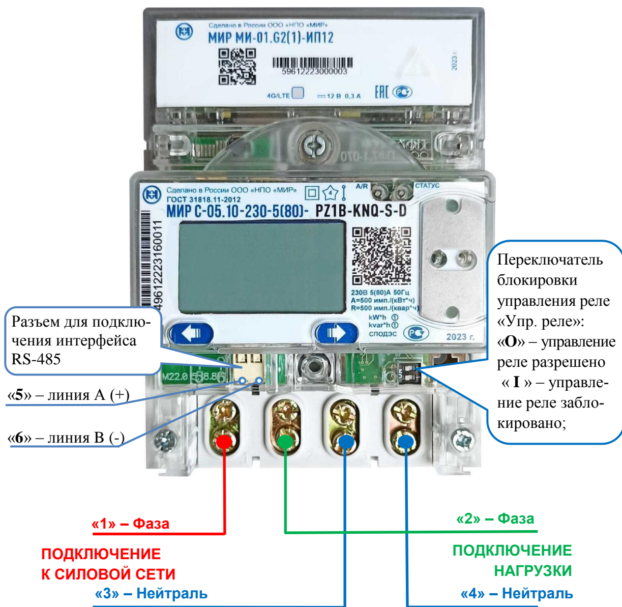
Рисунок Б.8 – Счетчик для установки на DIN-рейку со снятой крышкой зажимов
