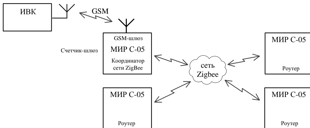
Рисунок 7.8 – Пример организации двухуровневой системы передачи данных с использованием сети ZigBee
