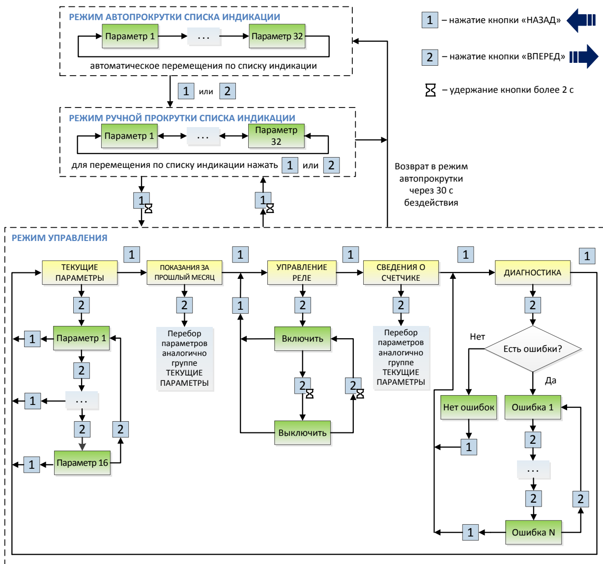
Рисунок 9.42 – Режимы индикации дисплея счетчика для установки на DIN-рейку
