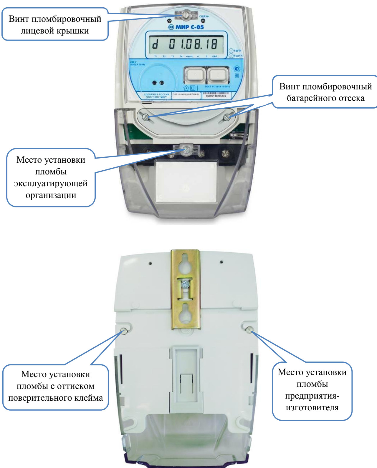
Рисунок 11.1 – Пломбирование счетчика для установки на щит
