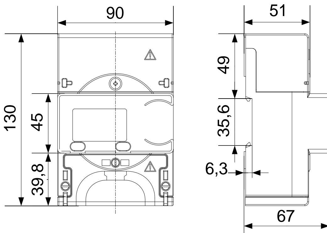
Рисунок Б.2 – Внешний вид, габаритные и установочные размеры счетчика внутренней установки для установки на DIN-рейку
