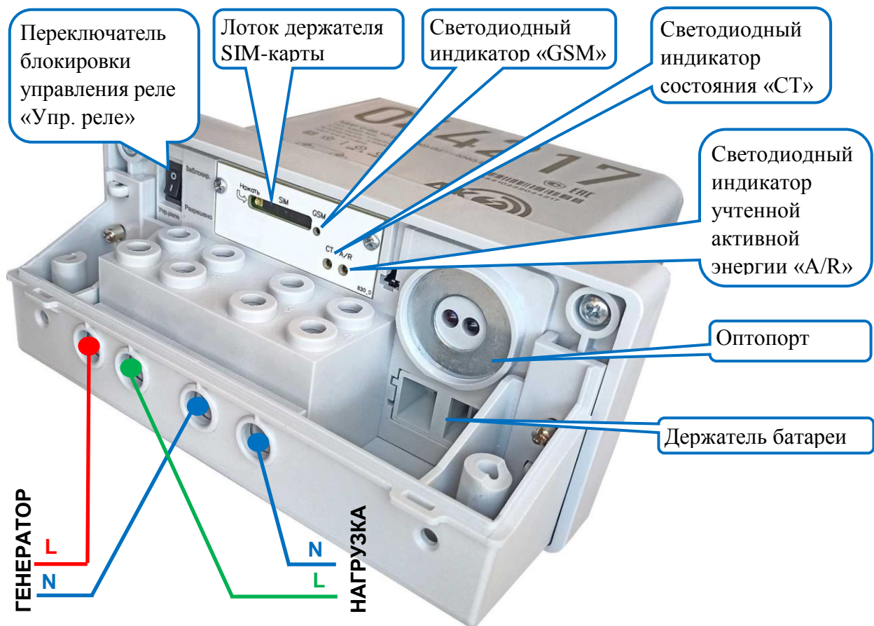
Рисунок Б.9 – Счетчик наружной установки с интерфейсом GSM со снятой крышкой зажимов (варианты исполнения контактной колодки с одним (сверху) и двумя (снизу) винтами на провод)
