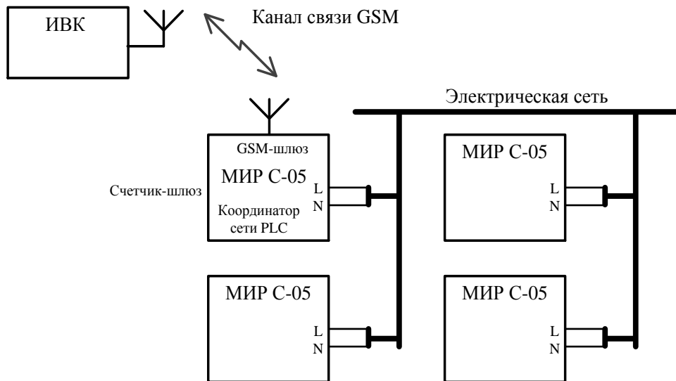
Рисунок 7.6 – Пример организации двухуровневой системы передачи данных с использованием сети PLC
