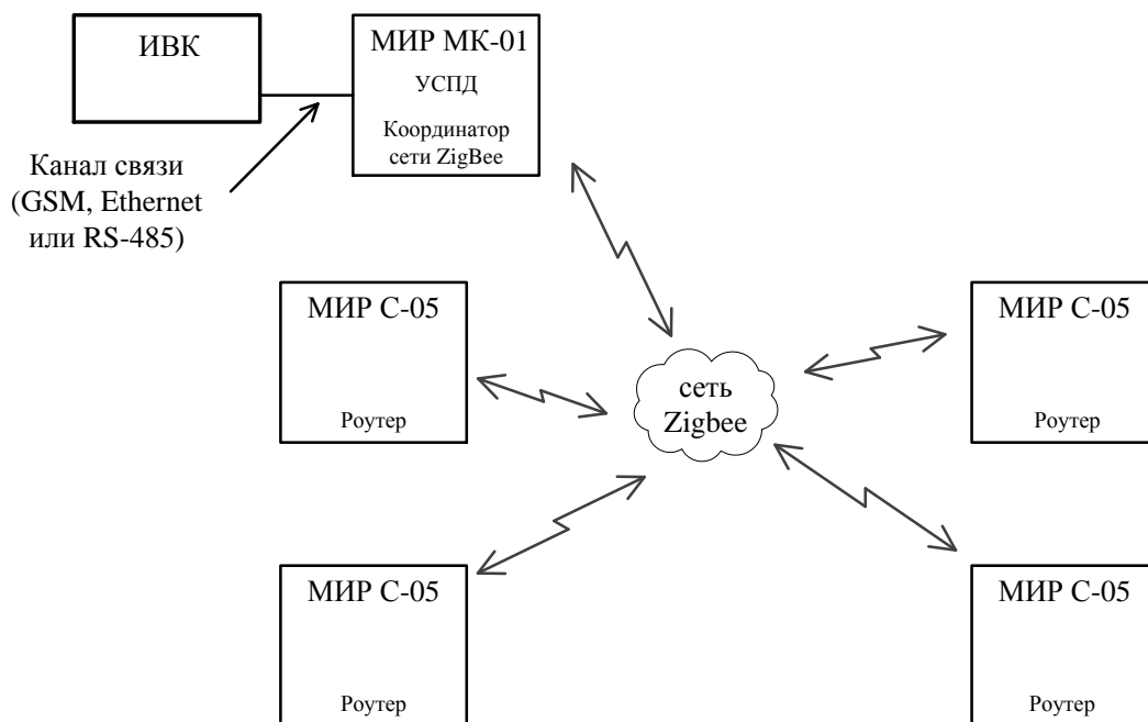
Рисунок 7.7 – Пример организации трехуровневой системы передачи данных с использованием сети ZigBee
