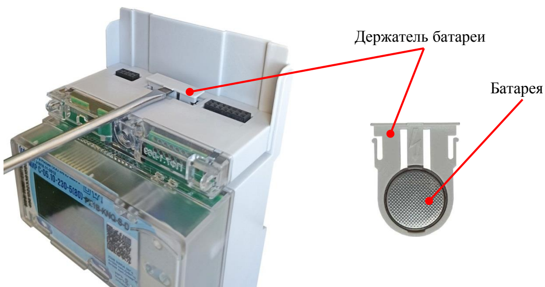
Рисунок 14.2 – Замена батареи в счетчике для установки на DIN-рейку
