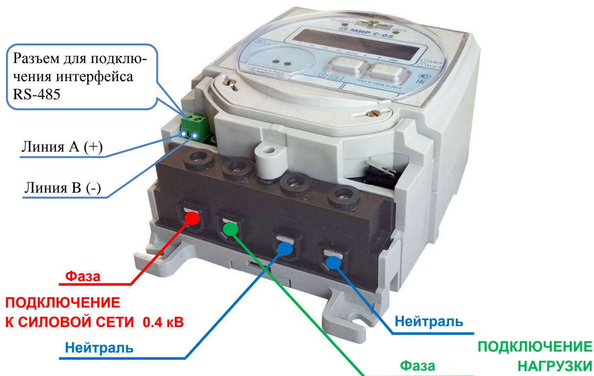
Рисунок Б.6 – Счетчик для установки на щит с интерфейсом RS-485 со снятой крышкой зажимов
