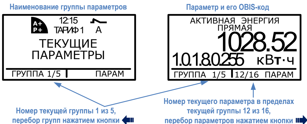
Рисунок 9.43 – Навигация по группам и параметрам в режиме управления счетчика для установки на DIN-рейку
