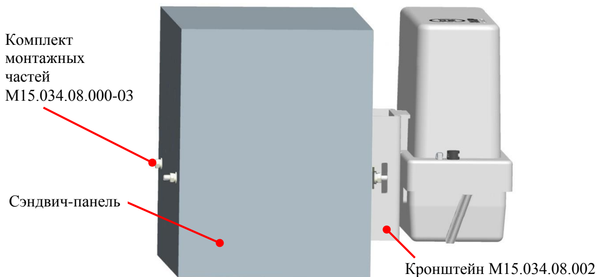
Рисунок 9.6 – Установка счетчика на сэндвич-панель
