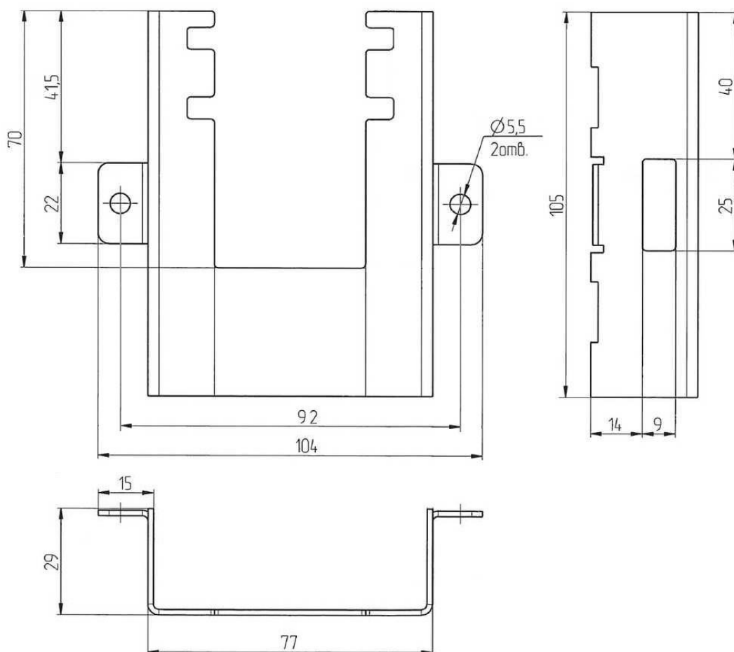
Рисунок Б.5 – Внешний вид, габаритные и установочные размеры кронштейна М15.034.08.002
