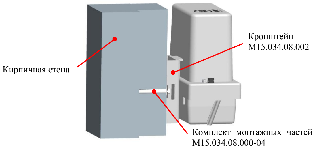
Рисунок 9.7 – Установка счетчика на кирпичную или бетонную стену здания
