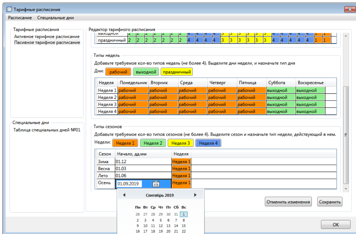
Рисунок 9.37 – Настройка недель в сезоне
