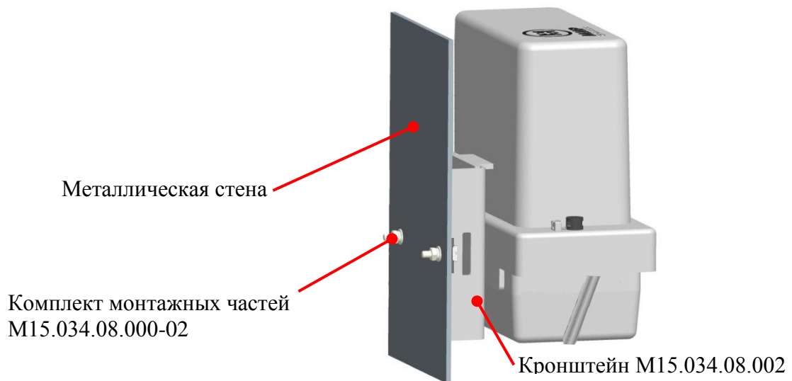
Рисунок 9.5 – Установка счетчика на металлическую стену
