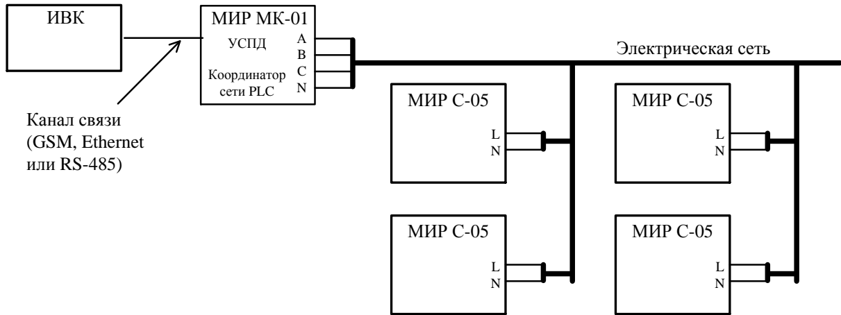
Рисунок 7.5 – Пример организации трехуровневой системы передачи данных с использованием сети PLC
