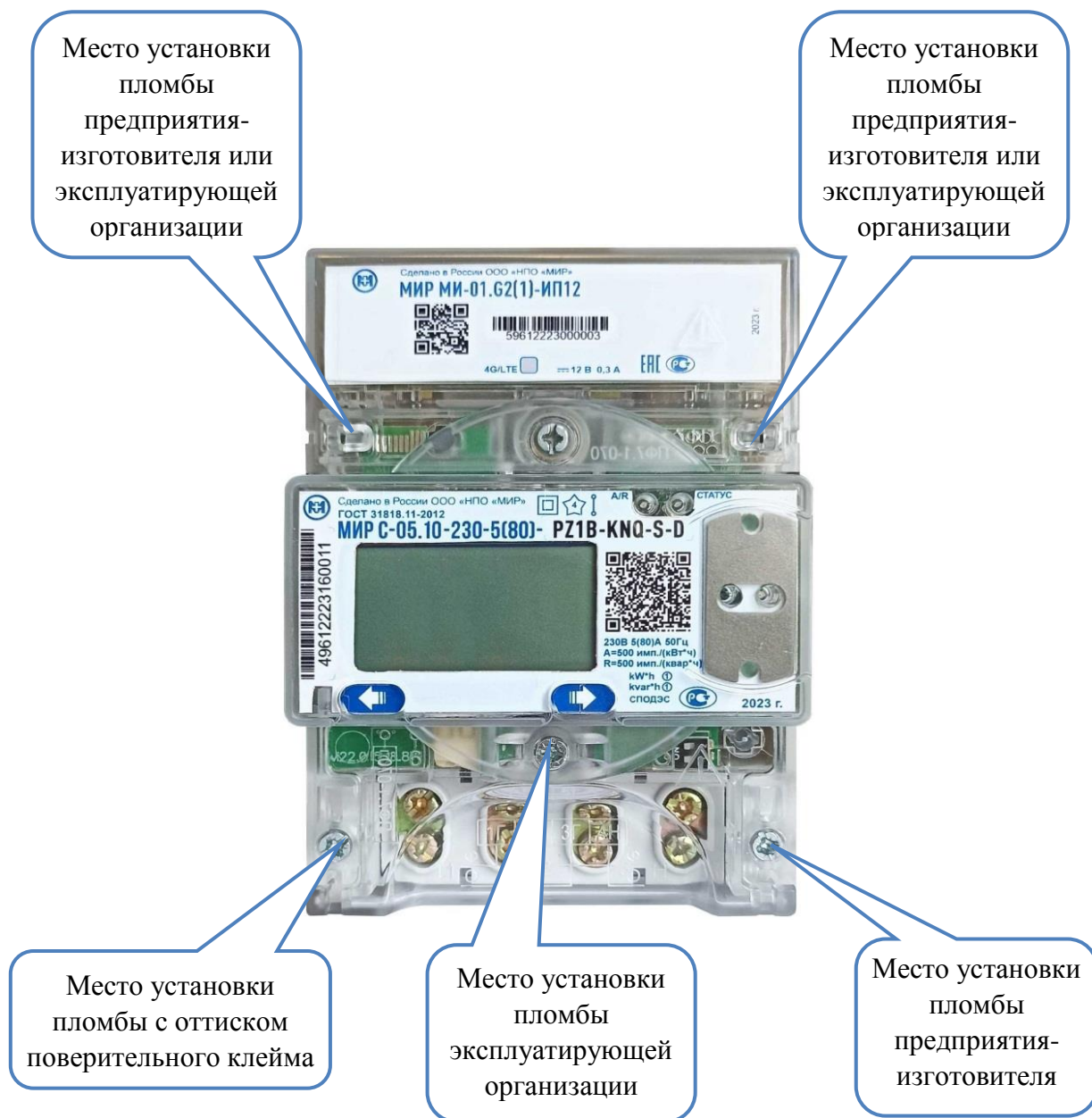
Рисунок 11.2 – Пломбирование счетчика для установки на DIN-рейку
