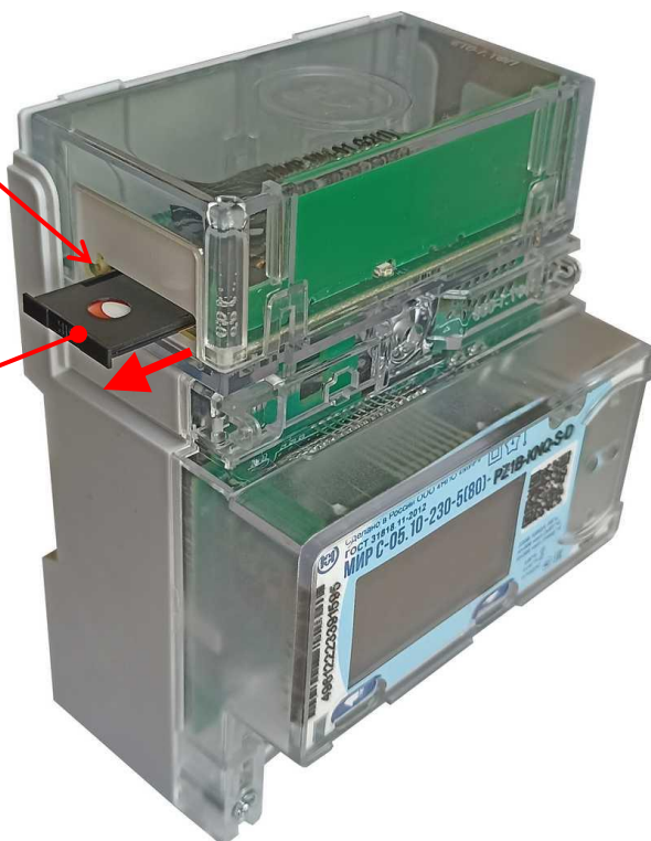
Рисунок 14.6 – Установка SIM-карты в счетчике для установки на DIN-рейку
