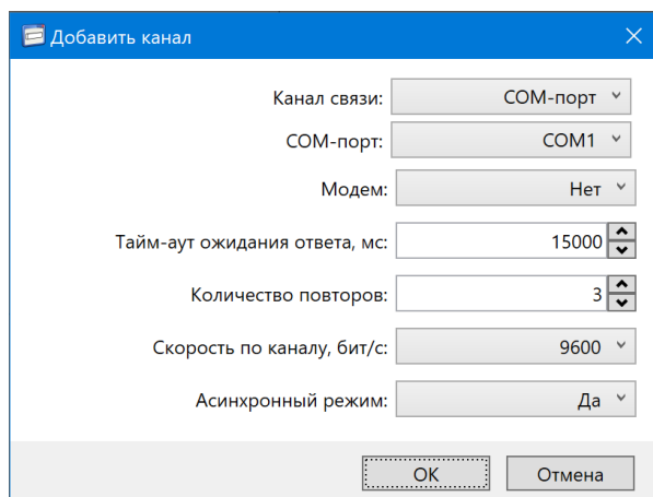
Рисунок 9.10 – Добавление канала связи со счетчиком
