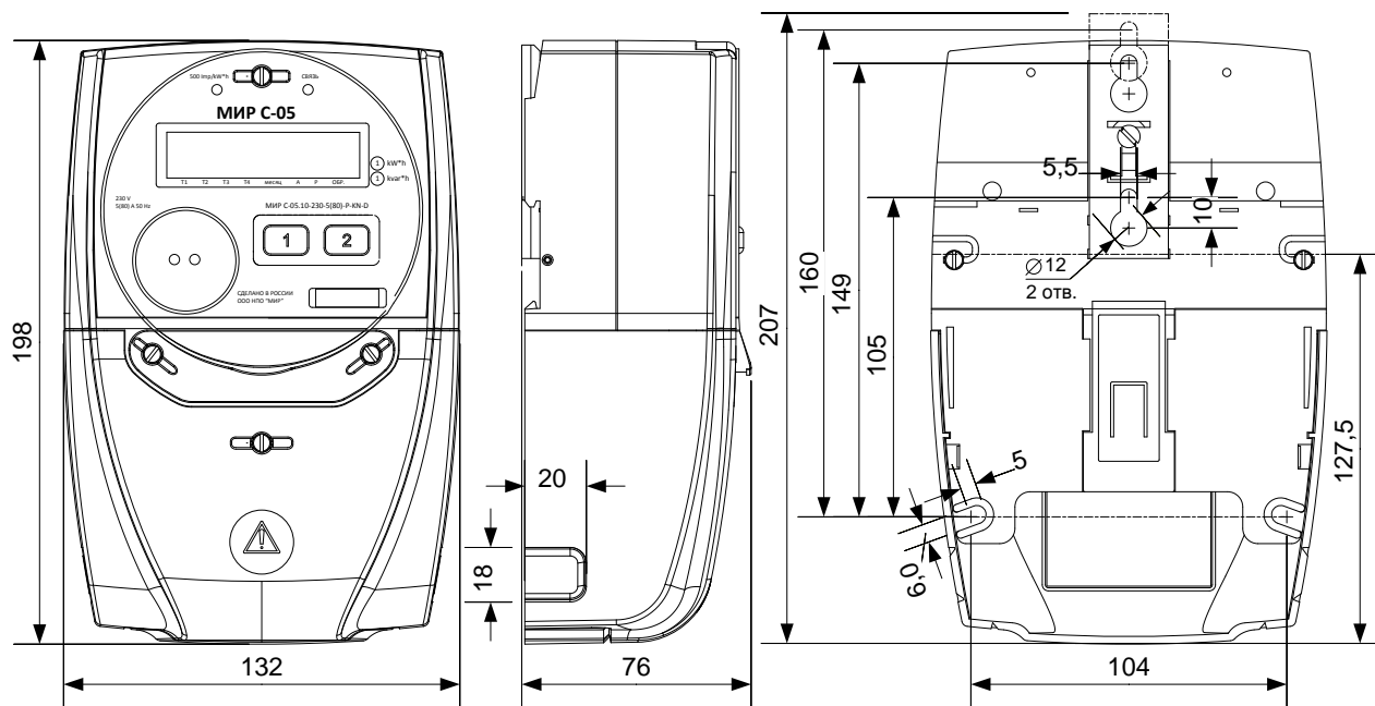
Рисунок Б.1 – Внешний вид, габаритные и установочные размеры счетчика внутренней установки для установки на щит
