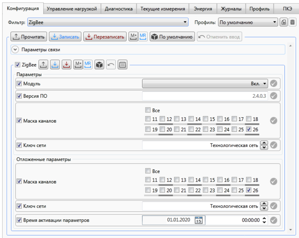
Рисунок 9.22 – Настройка параметров интерфейса ZigBee счетчика
