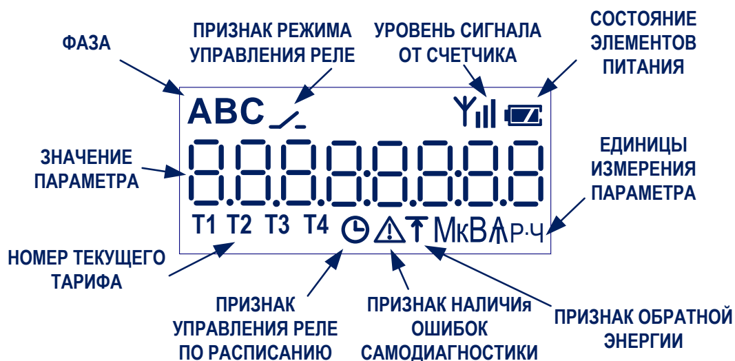
Рисунок 4.1 – Внешний вид и назначение сегментов индикатора дисплея
