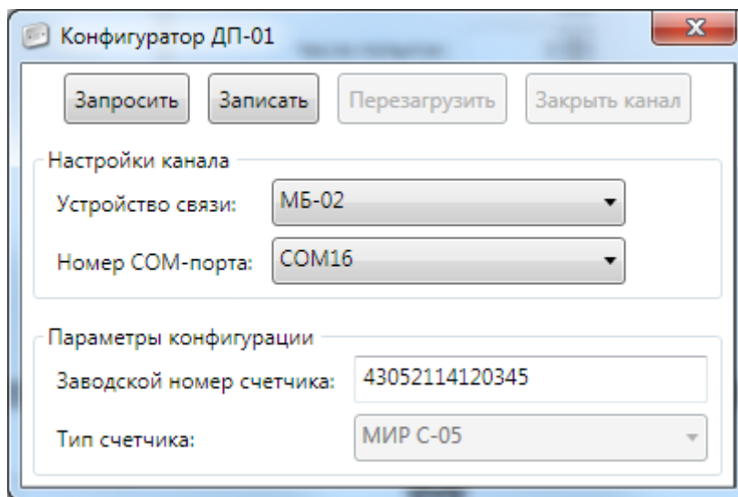
Рисунок 4.6 – Конфигурирование ДП-01
