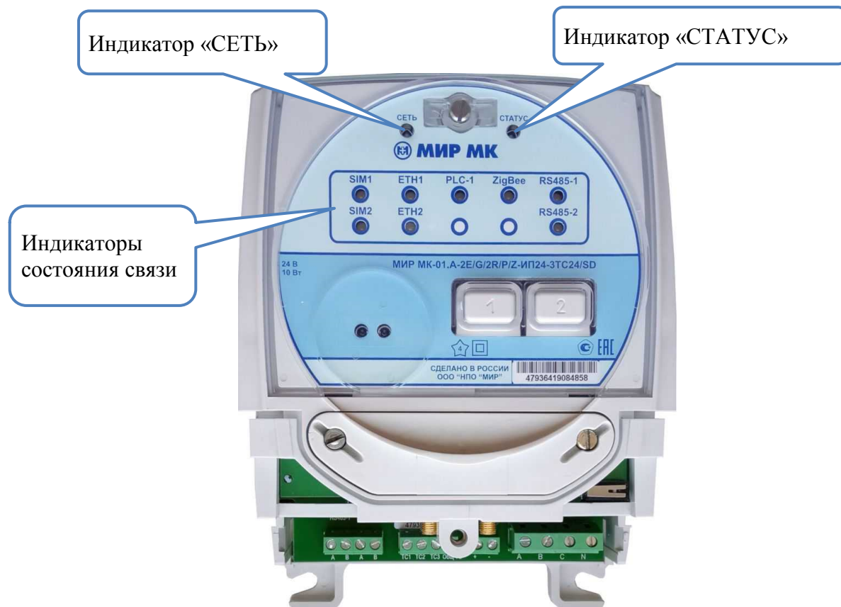
Рисунок 5.3 – Расположение индикаторов коммуникатора МИР МК-01.А-2E/G/2R/P/Z-ИП24-3ТС24/SD
