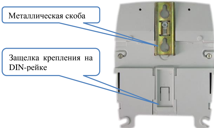
Рисунок 5.4 – Элементы крепления коммуникатора
