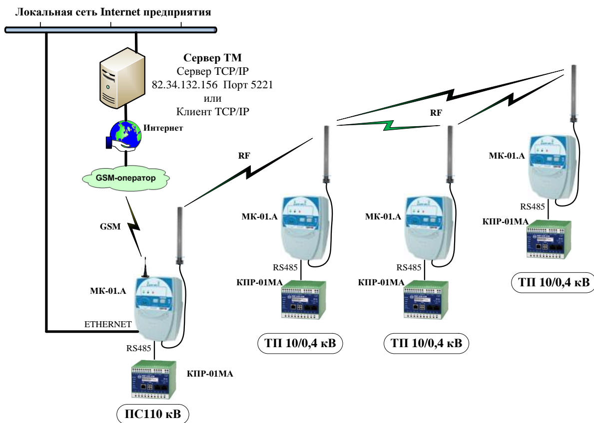
Рисунок 8.48 – Пример использования коммуникатора с интерфейсом GSM в качестве каналообразующего оборудования для ЦРЭС
