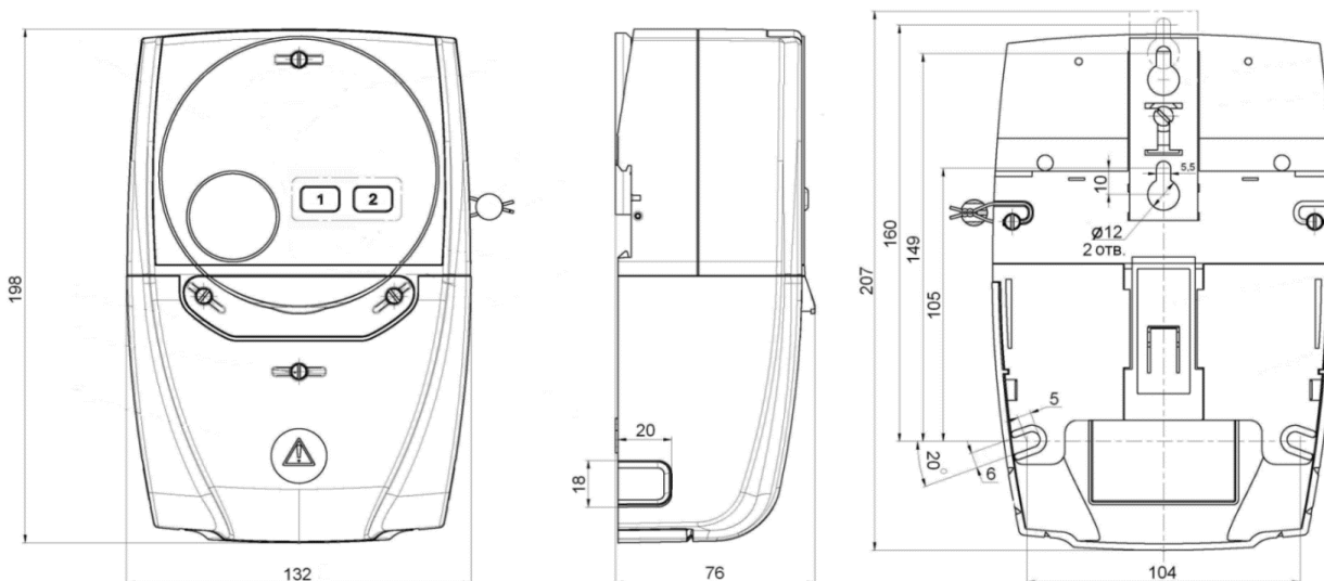
Рисунок 2.1 – Габаритные и установочные размеры коммутатора
