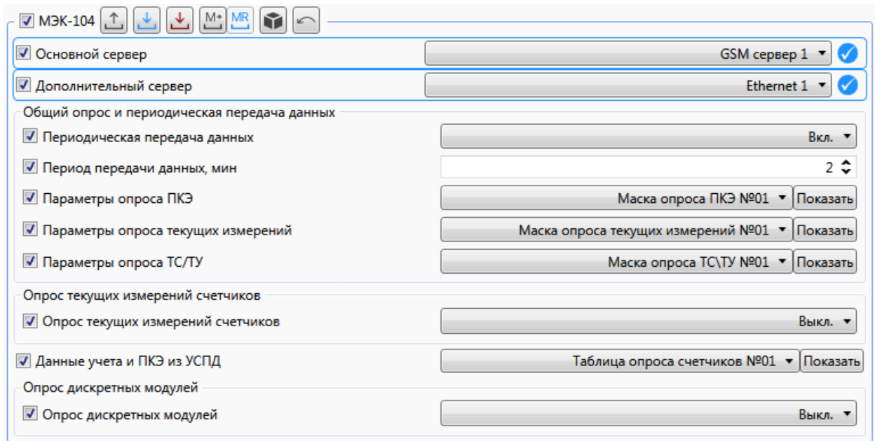
Рисунок 8.31 – Окно выбора таблиц параметров, порогов опроса и данных учета и ПКЭ
