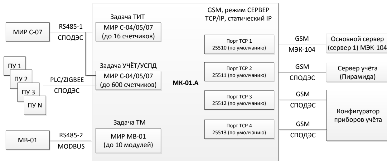
Рисунок 8.51 – Типовая схема включения коммутатора по протоколу МЭК-104
