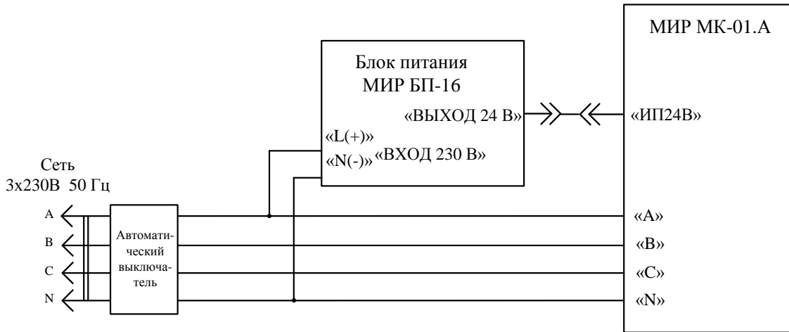
Рисунок А.1 – Схема подключения питания коммутатора с использованием ионисторного блока питания МИР БП-16
