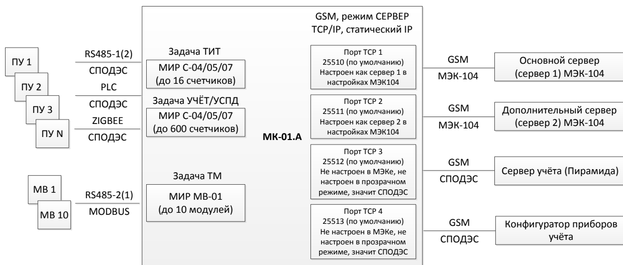
Рисунок 8.50 – Структурная схема использования коммутатора по протоколу МЭК-104
