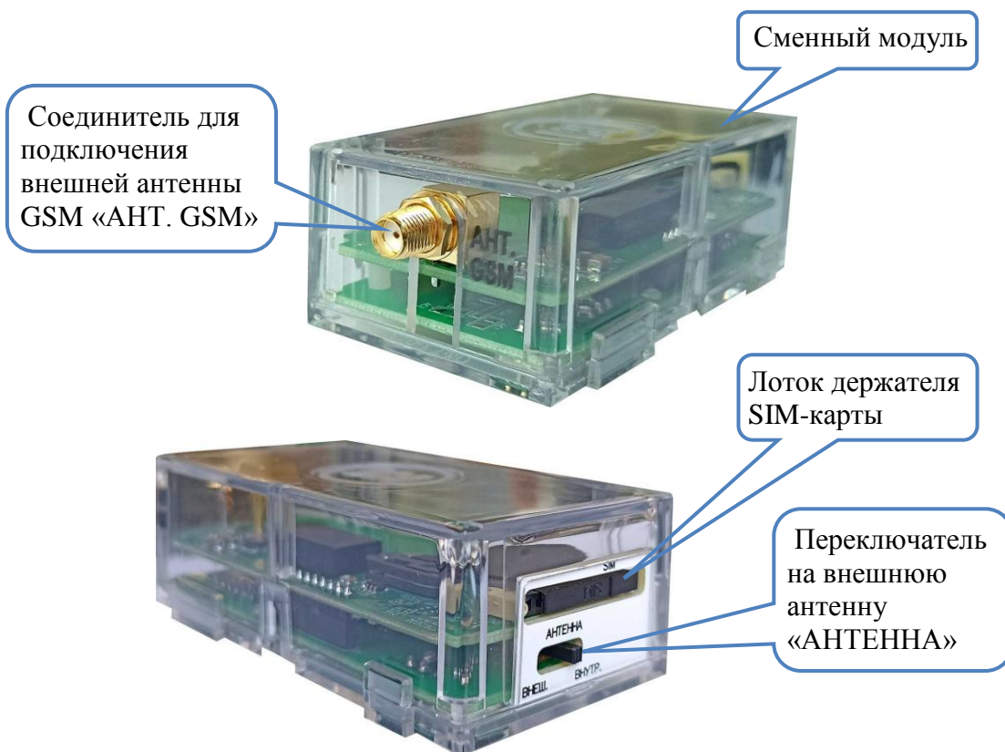
Рисунок Б.3 – Внешний вид, габаритные и установочные размеры сменного модуля счетчика для установки на DIN-рейку (приведен внешний вид сменного модуля с возможностью подключения внешней антенны)
