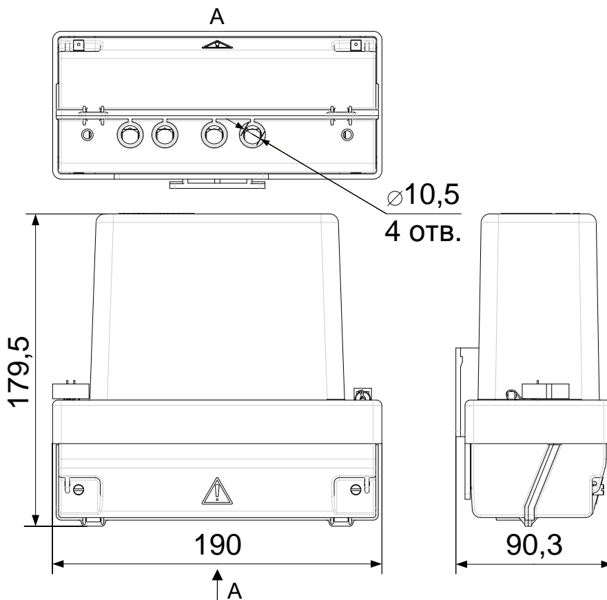
Рисунок Б.4 – Внешний вид, габаритные и установочные размеры счетчика
