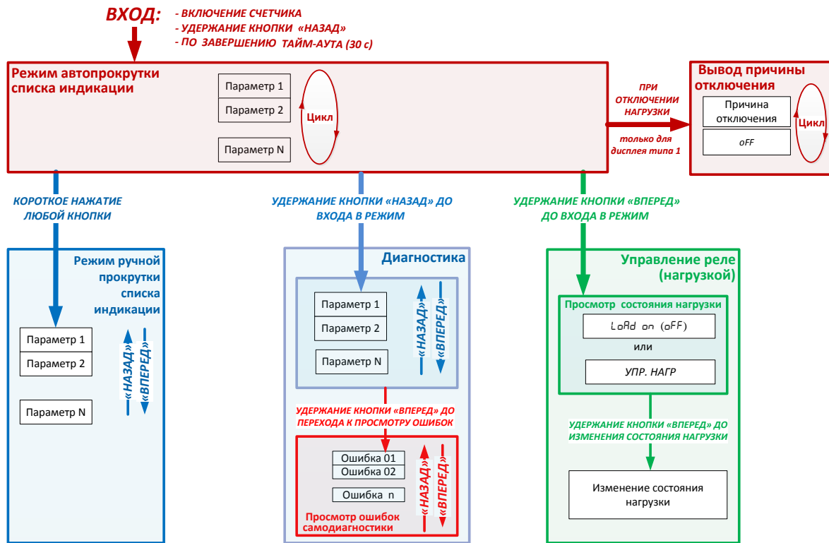
Рисунок 9.41 – Режимы индикации дисплея счетчика для установки на щит
