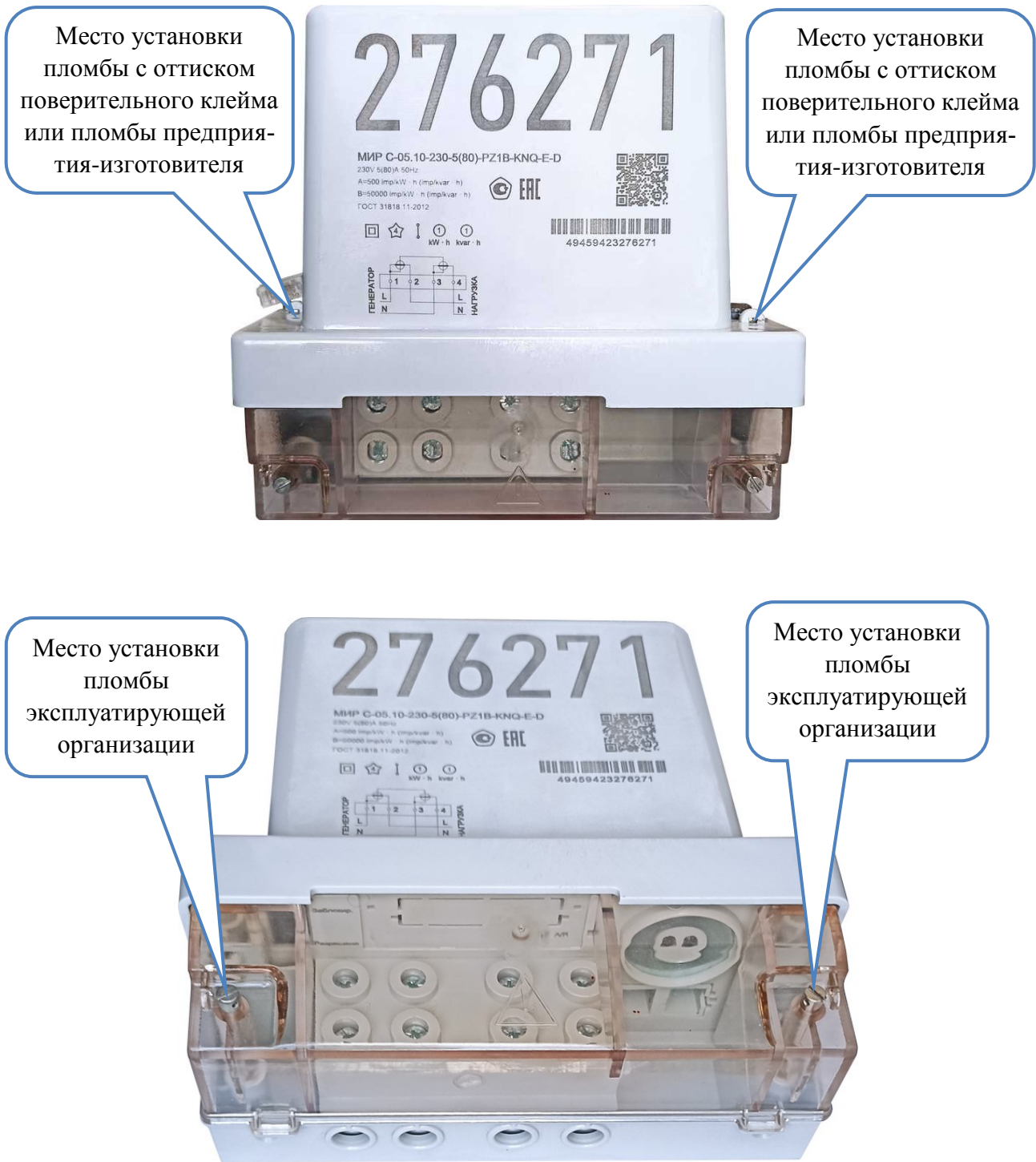
Рисунок 11.3 – Пломбирование счетчика наружной установки
