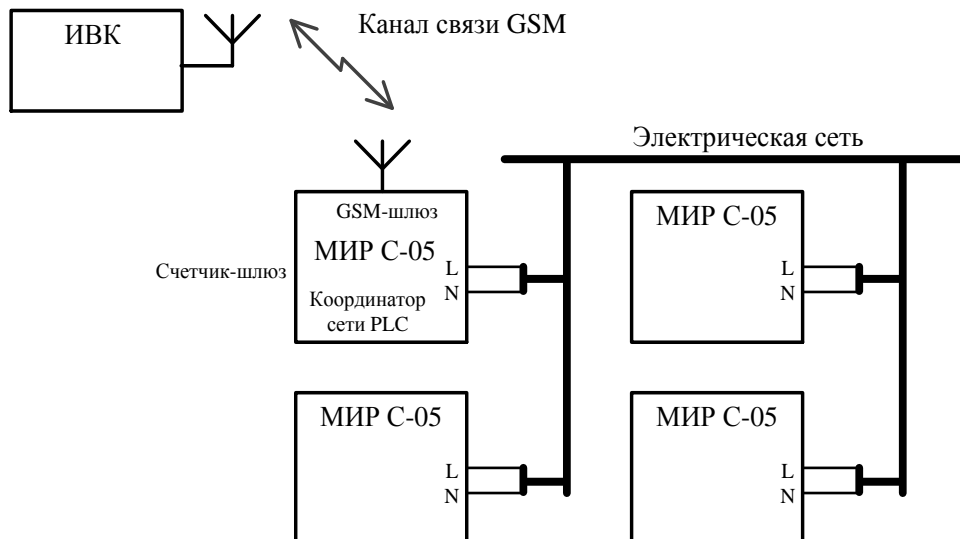
Рисунок 7.6 – Пример организации двухуровневой системы передачи данных с использованием сети PLC
