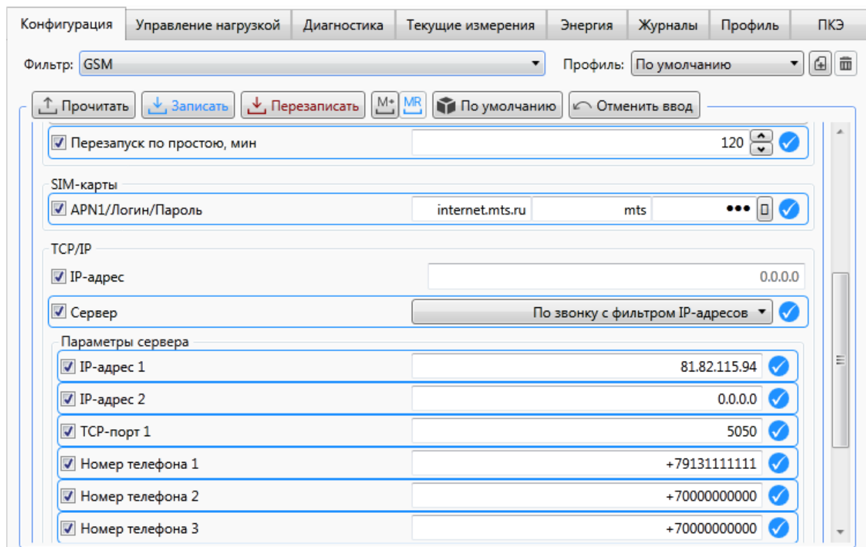
Рисунок 9.24 – Настройка параметров счетчика в качестве сервера TCP/IP
